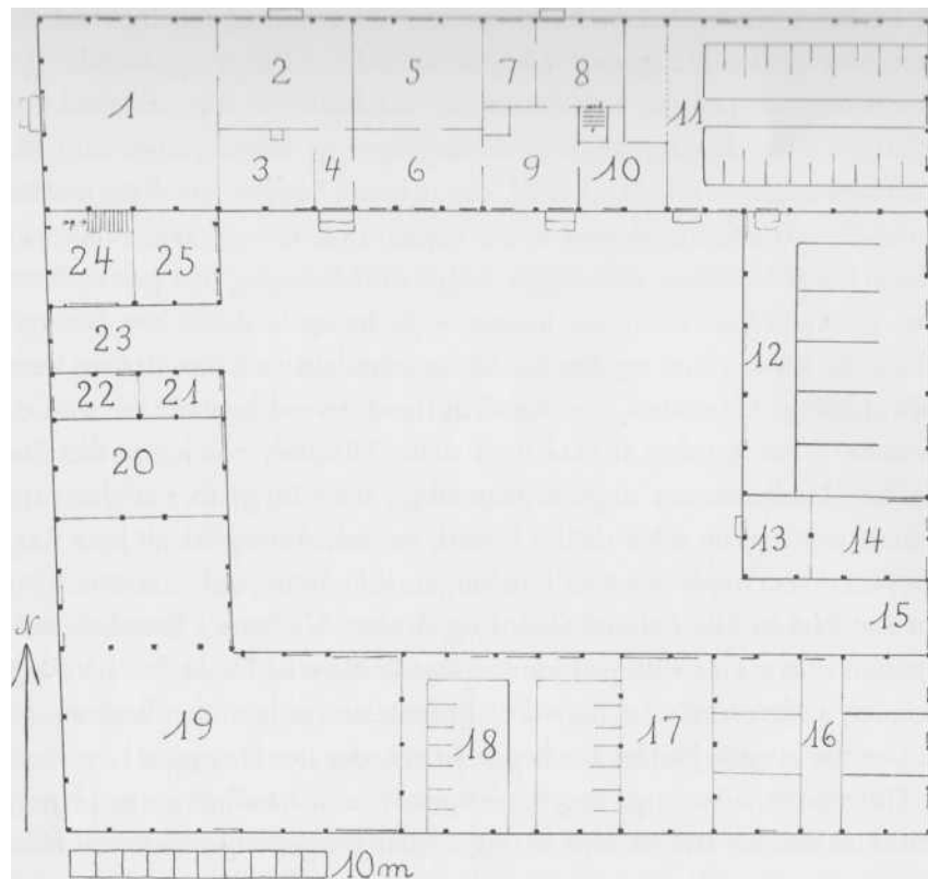
Plan over Jens Rasmussens gård, bygget 1793—95, opmålt og tegnet af forf.
